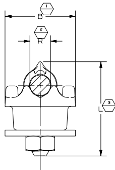
VIEW A-A
